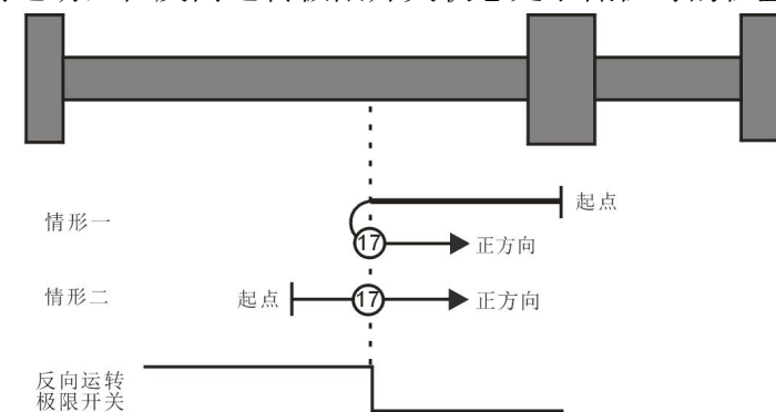
取决于反向运转极限开关的原点回零，上图中的表示①7原点回零模式17
