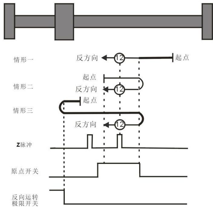
取决于原点开关、反向运转极限开关和Z脉冲的原点回零，上图中的表示⑫原点回零模式12
