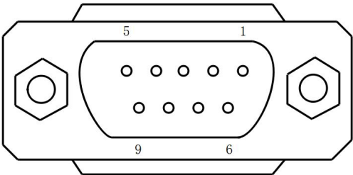
9pin 引脚接口（母头）
