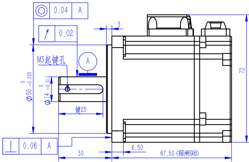
电机技术规格 Motor specifications
